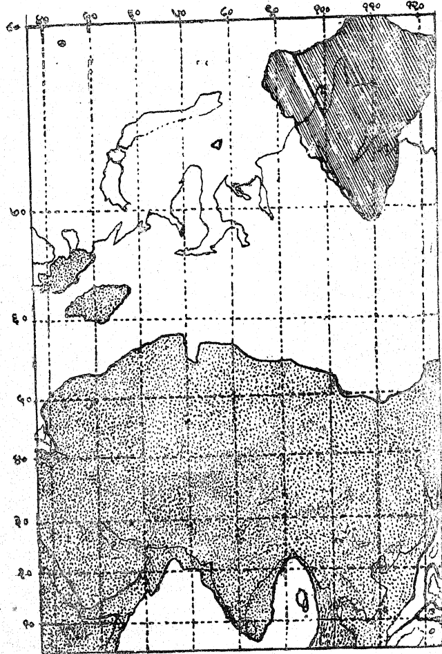
चित्र ४६—जंबू द्वीप, दस लाख से आठ लाख वर्ष पूर्व तक अंशकार की कृपा ] [ वेद-काल-निर्णय से
